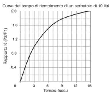
Curva di riempimento
