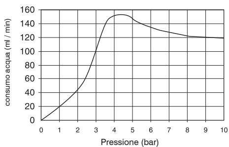
Curva consumo acqua
