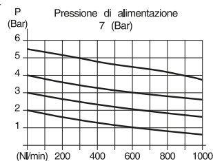
CURVE DI PORTATA DA 1 A 2
