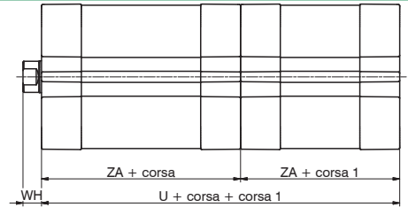
In spinta steli indipendenti
