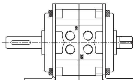
Montaggio con flange
