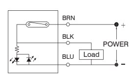
con ampolla Reed, 3 fili
