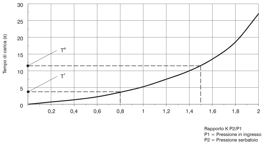
Caratteristiche di riempimento (serbatoio 5 litri)
