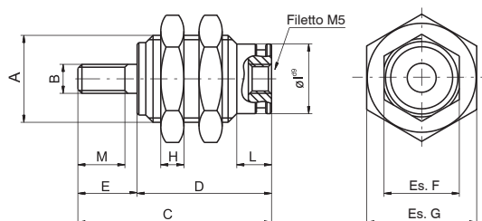
Semplice effetto molla anteriore stelo filettato
