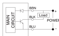
ad effetto Hall-NPN, 3 fili
