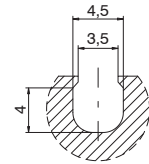
Particolare Cava tipo "D" per Sensore
