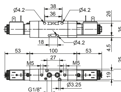
Peso 290 g Pressione minima di funzionamento 2 bar
