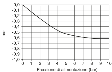
Curva vuoto generato
