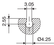
Particolare cava tipo "C" per sensore
