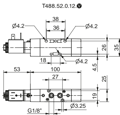
Peso 190 g Pressione minima di funzionamento 2,5 bar
