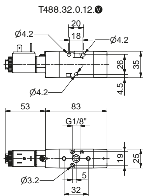
Peso 160 g Pressione minima di funzionamento 2,5 bar
