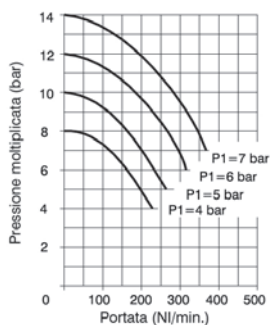
Diagramma delle portate
