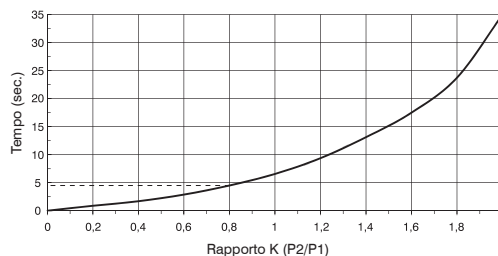
Curva del tempo di riempimento di un serbatoio di 5 litri
