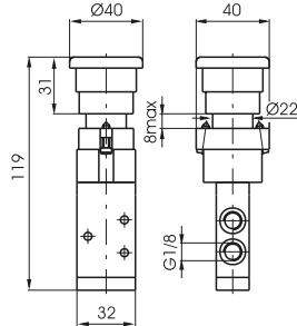
Peso 235 g Forza di azionamento 33 N
