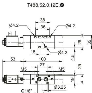
Peso 190 g Pressione minima di funzionamento 2,5 bar
