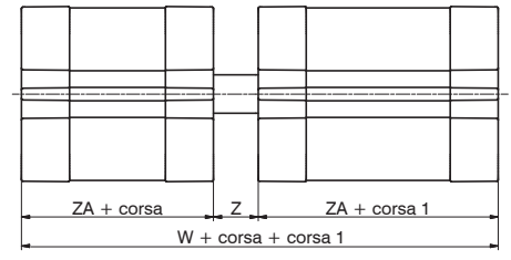
Contrapposti stelo comune
